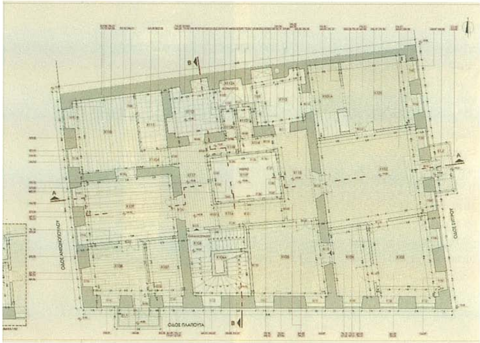
Εικ. 8. Κτίριο Άρμανσπεργκ – κάτοψη α' ορόφου – αποτύπωση..
