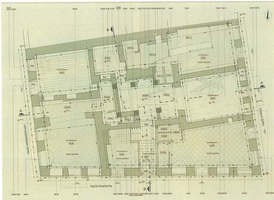
Εικ. 2. Κτίριο Αρμανσμπεργκ: Κάτοψη στάθμης ισογείου – αποτύπωση.
