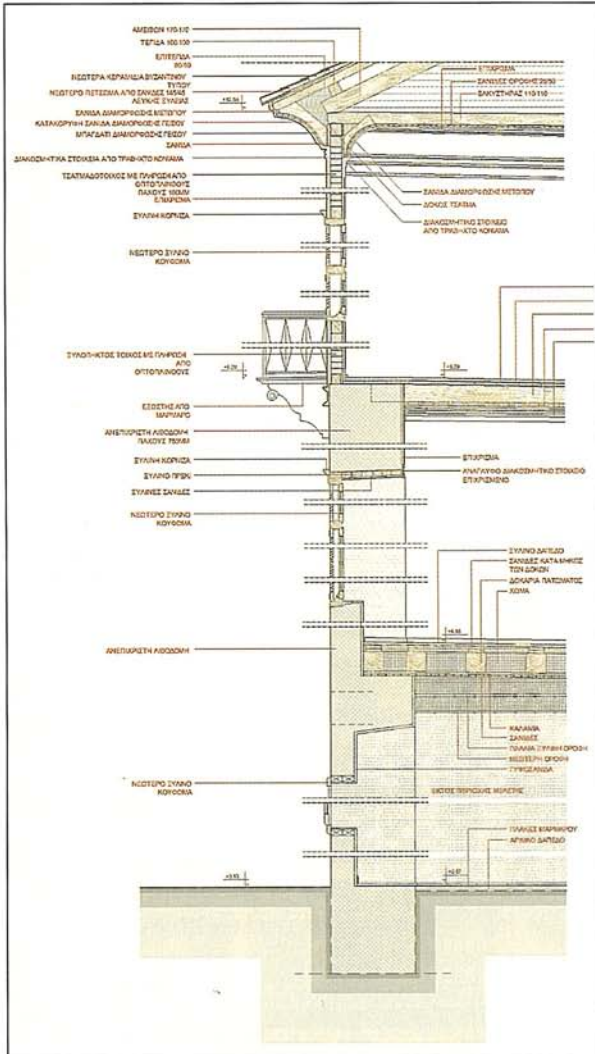
Εκ. 17. Κατασκευαστική τομή του κτιρίου.
