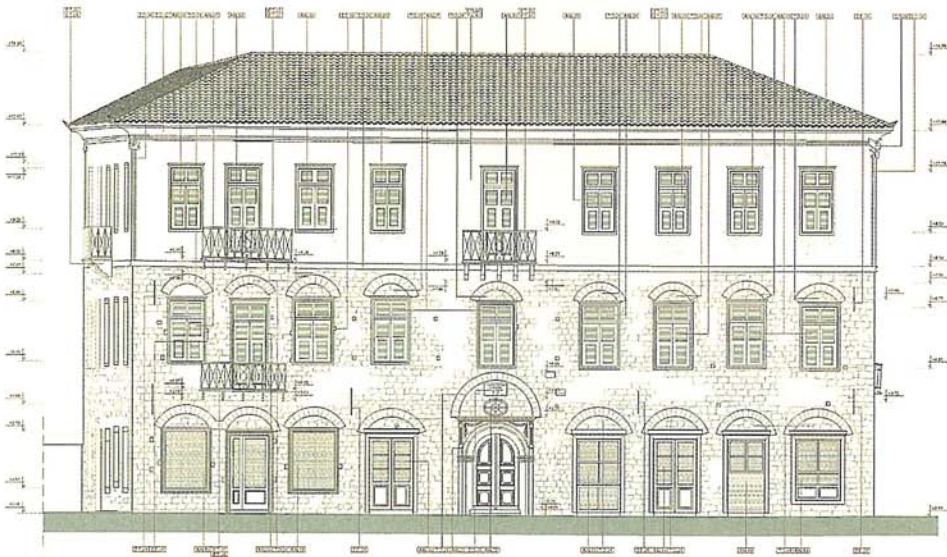
Εικ. 16. Κτίριο Άρμανσπεργκ – δυτική όψη – αποτύπωση.
