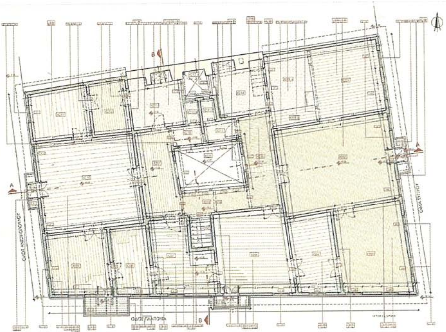
Εικ. 11. Κτίριο Άρμανσπεργκ – κάτοψη β' ορόφου.
