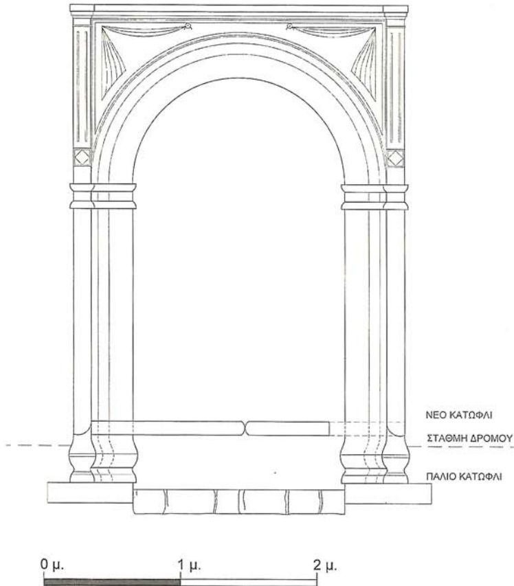
Εικόνα 1: Η πόρτα της οικίας Άρμανσπεργκ.
